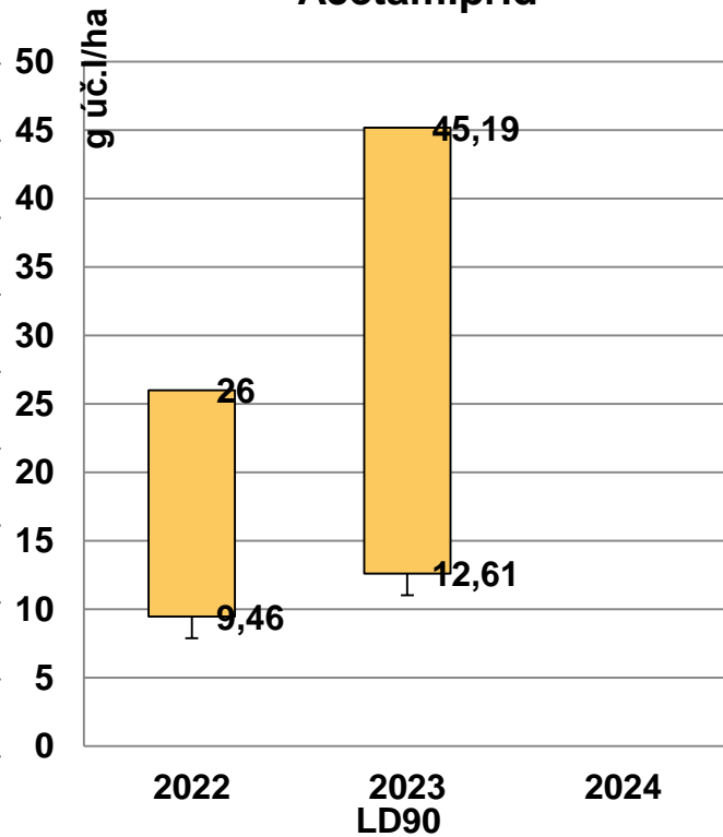
Acetamiprid
