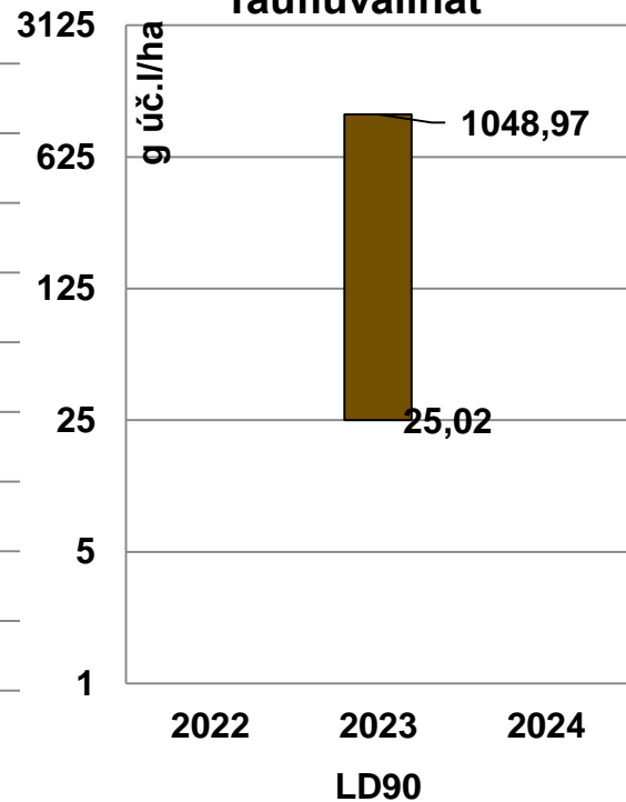
Taufluvalinát
